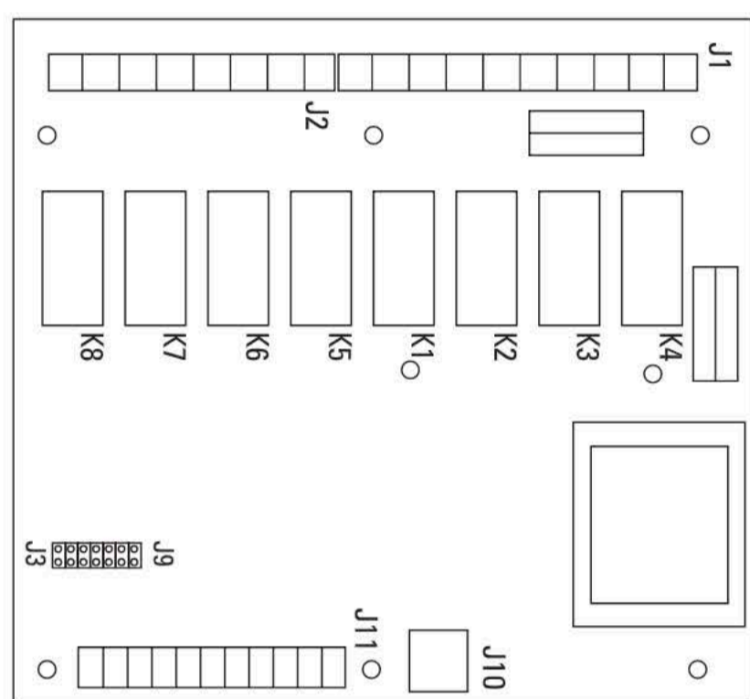
Oikosulkupalat
