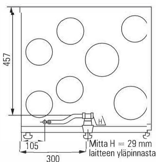
ILTO 450 Econon putkiliitäntä
